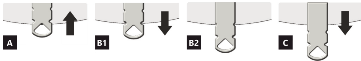
Abb. 9 Luftzufuhrregler – Typ 5
