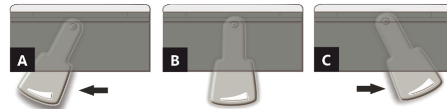
Abb. 6 Luftzufuhrregler – Typ 2
