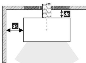
Hinterer Rauchrohranschluss
