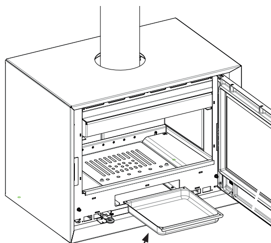
1 - TIROIR DE COLLECTE DES CENDRES
